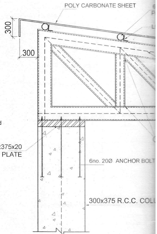
SECTION - Y - Y
